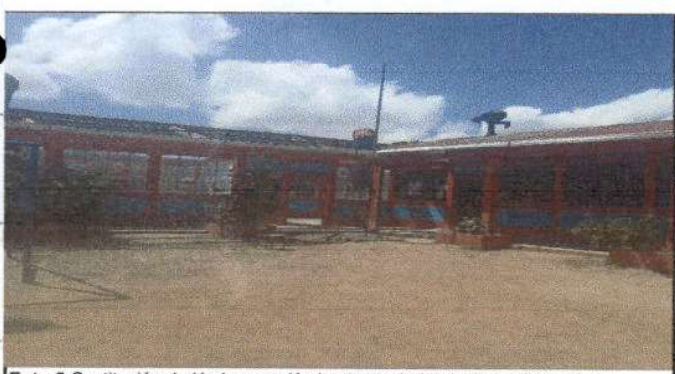
Foto 5: Sustitución de lámina, por lámina troquelada aluzinc calibre 26 y sustitución de bajada de agua pluvial de metal por tubo PVC 3".
